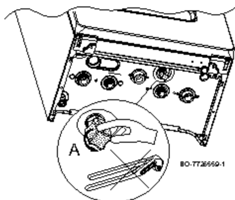
SI.142 Punjenje instalacije
