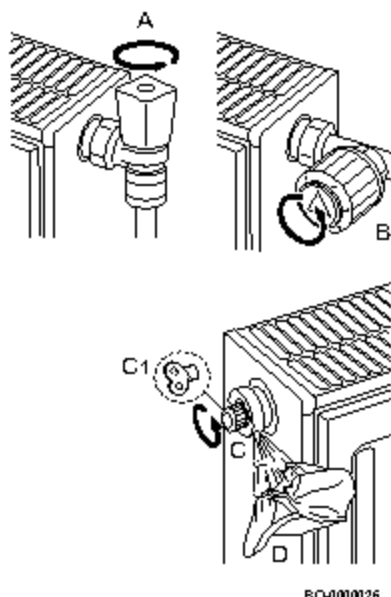
SI.106 Pročišćavanje instalacije
