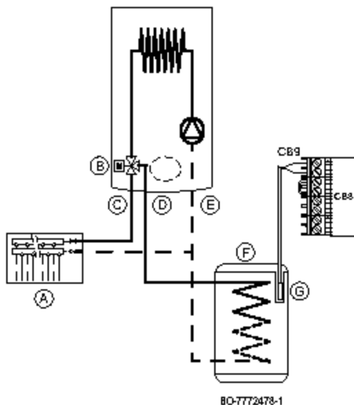
SI.120 Priključak rezervoara za TPV
