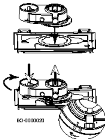
SI.127 Instaliranje razdvojenih cevi
