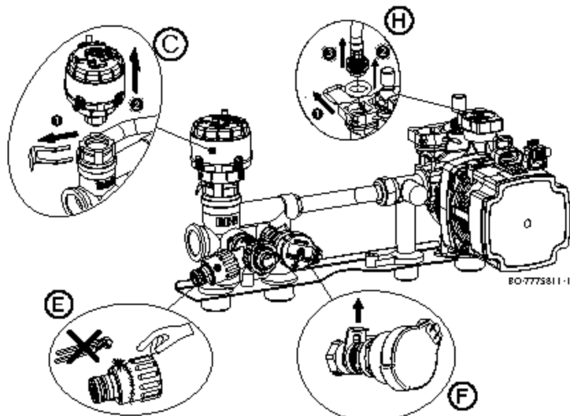
SI.165 Deo za jedinicu za vodu kotla namenjenog samo za grejanje, koja je unapred opremljena za povezivanje sa cilindrom TPV
