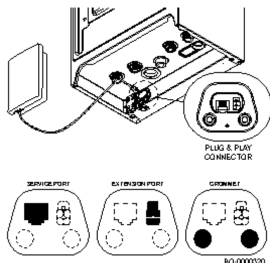
SI.133 Položaj konektora
