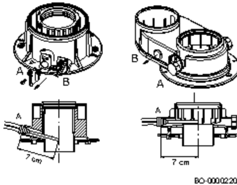
SI.147 Tipovi priključaka – merna tačka dimnog gasa
