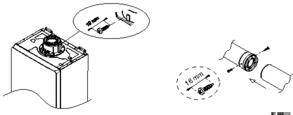
SI.124 Pričvrščivanje koaksijalnog tornja za otpadni gas
