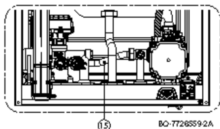
SI.111 Opis jedinice za vodu u modelu namenjenom samo za grejanje
