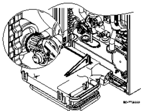
SI.143 Pražnjenje instalacija
