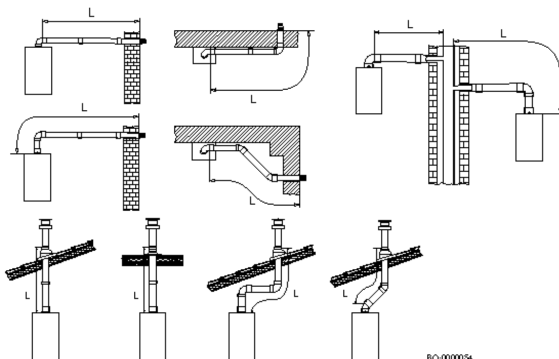
SI.125 Primeri instalacije koncentrične cevi
