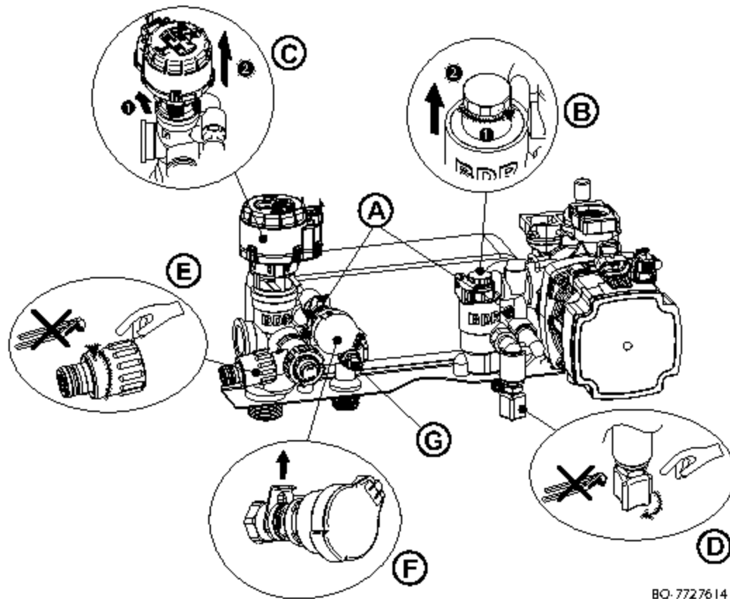
SI.164 Deo za grejanje + jedinica za vodu kombinovanog kotla za TPV
