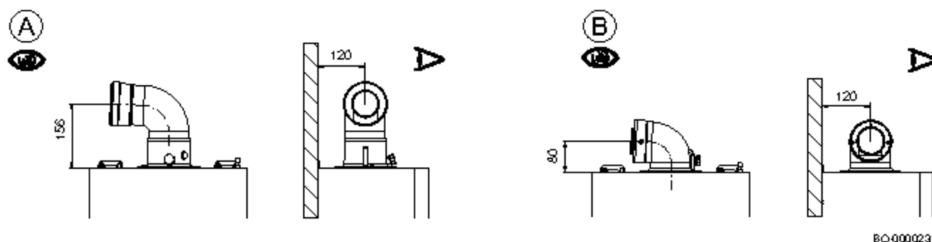
SI.123 Koncentrični tip za odvod-dovod
