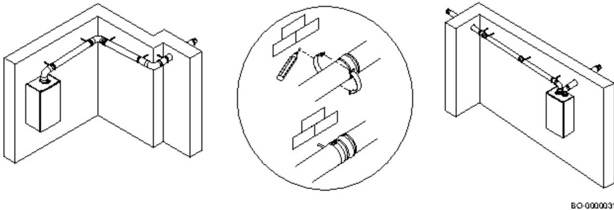
SI.121 Način pričvršćivanja cevi na zid
